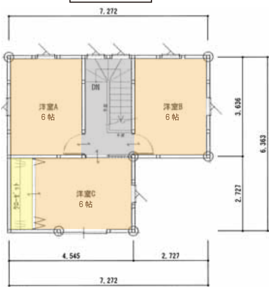
2F 平面図
